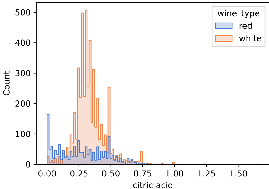
Histograma Incondicional (Bimodalidade) - citric acid
